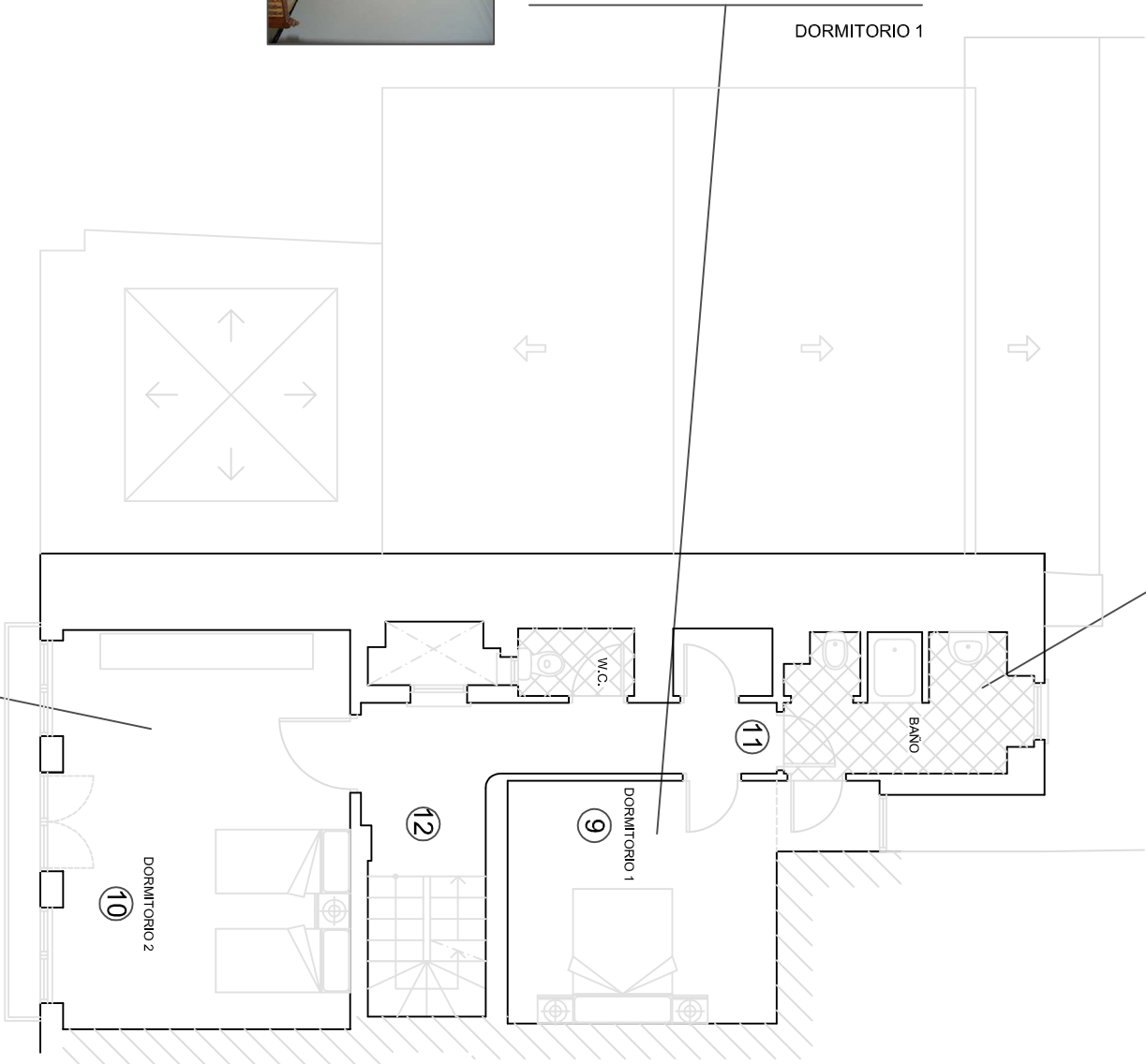
PLANTA SEGUNDA
